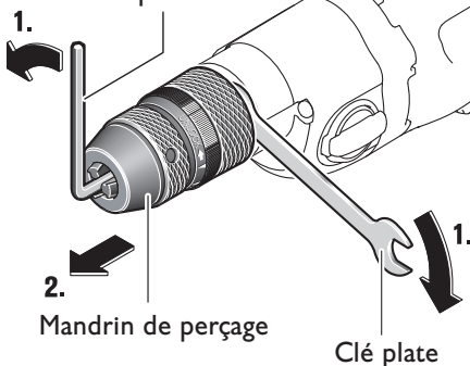
Fig. 3 Clé mâle coudée pour vis à six pans creux
